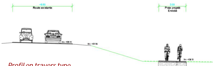
Profil en travers type
